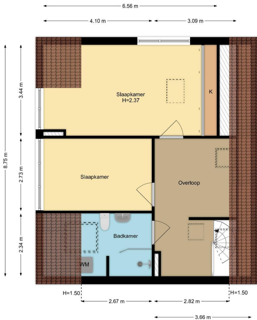
1e Verdieping Zonnegaarde 73, Zoeterwoude
